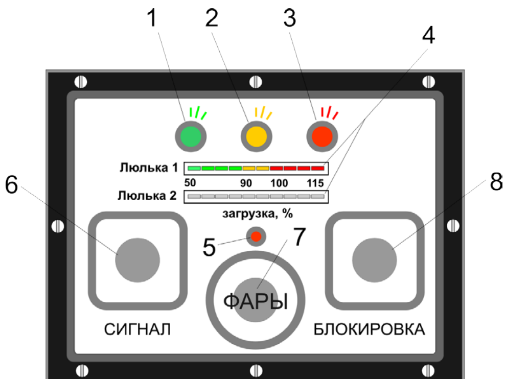
Рис. П1.2. Завершение настройки Люльки 1
