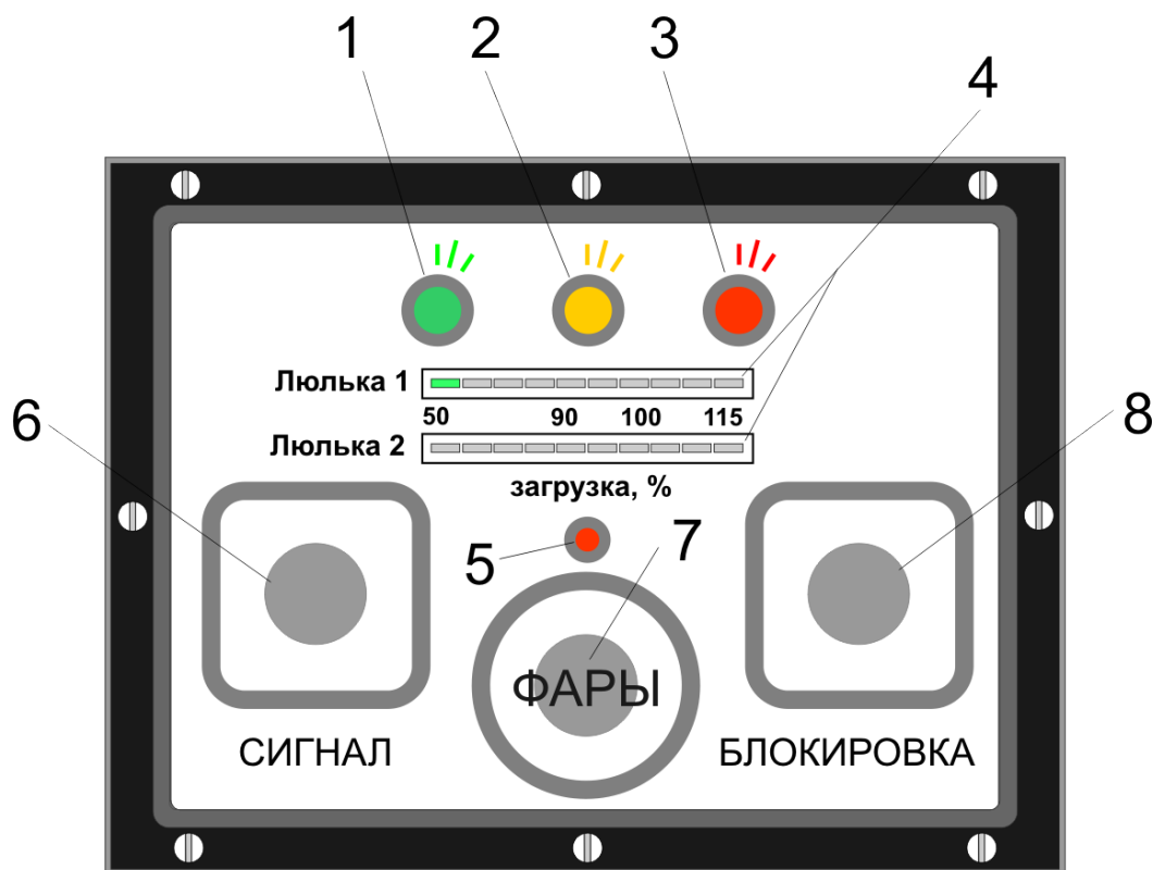
Рис.П1.1. Режим настройки первой люльки
