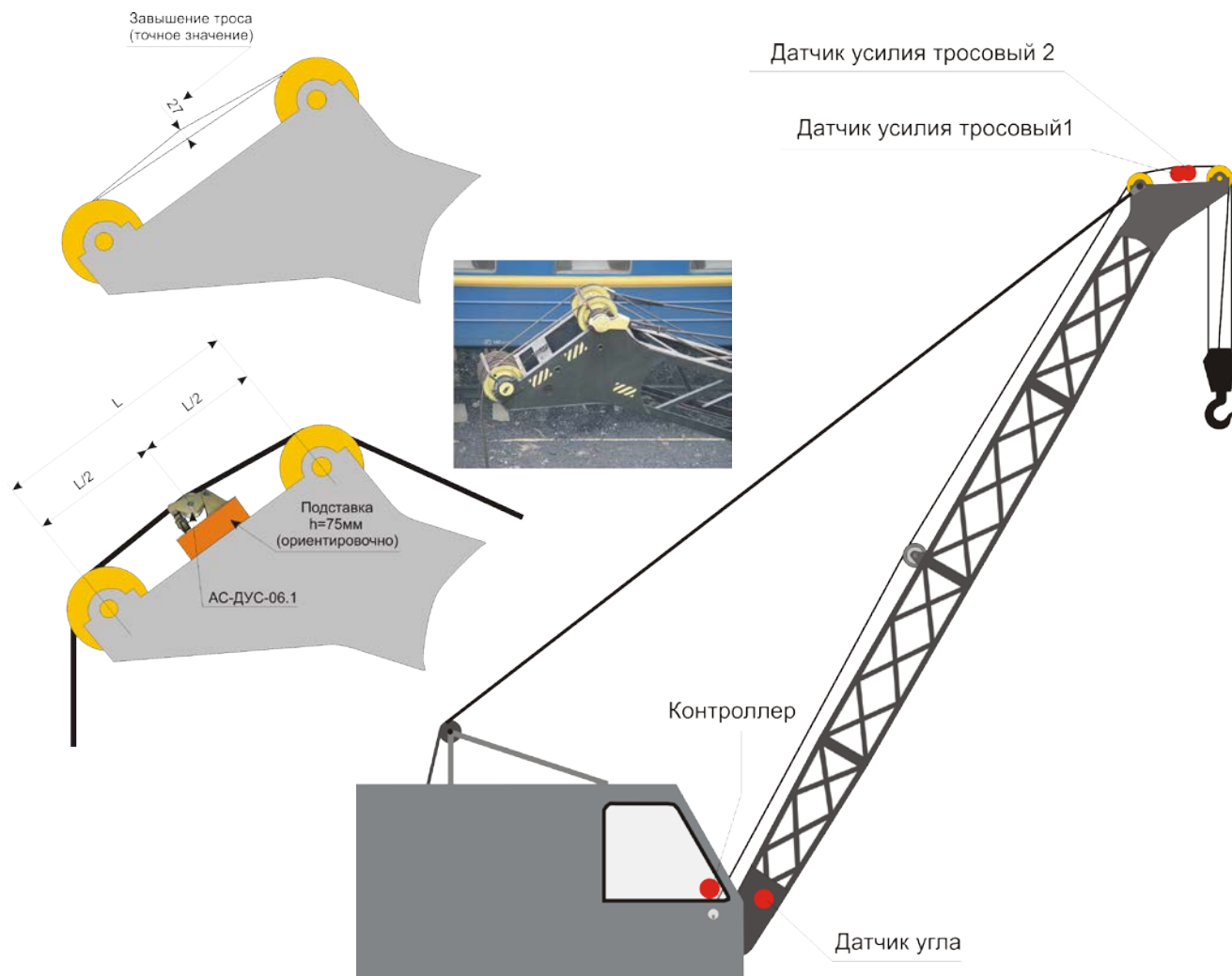
Рис.1 Система АС-АОГ-01м+ и ее размещение на кране
