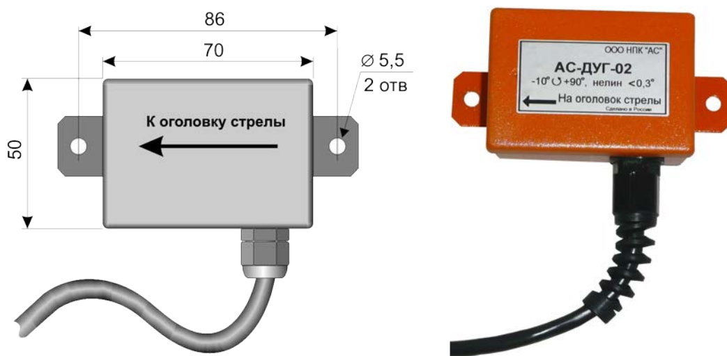
Рис. 6 Датчик угла системы АС-АОГ-01м+
