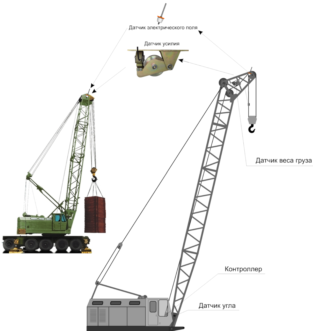
Рис.1 Система АС-АОГ-01м+ и ее размещение на кране
