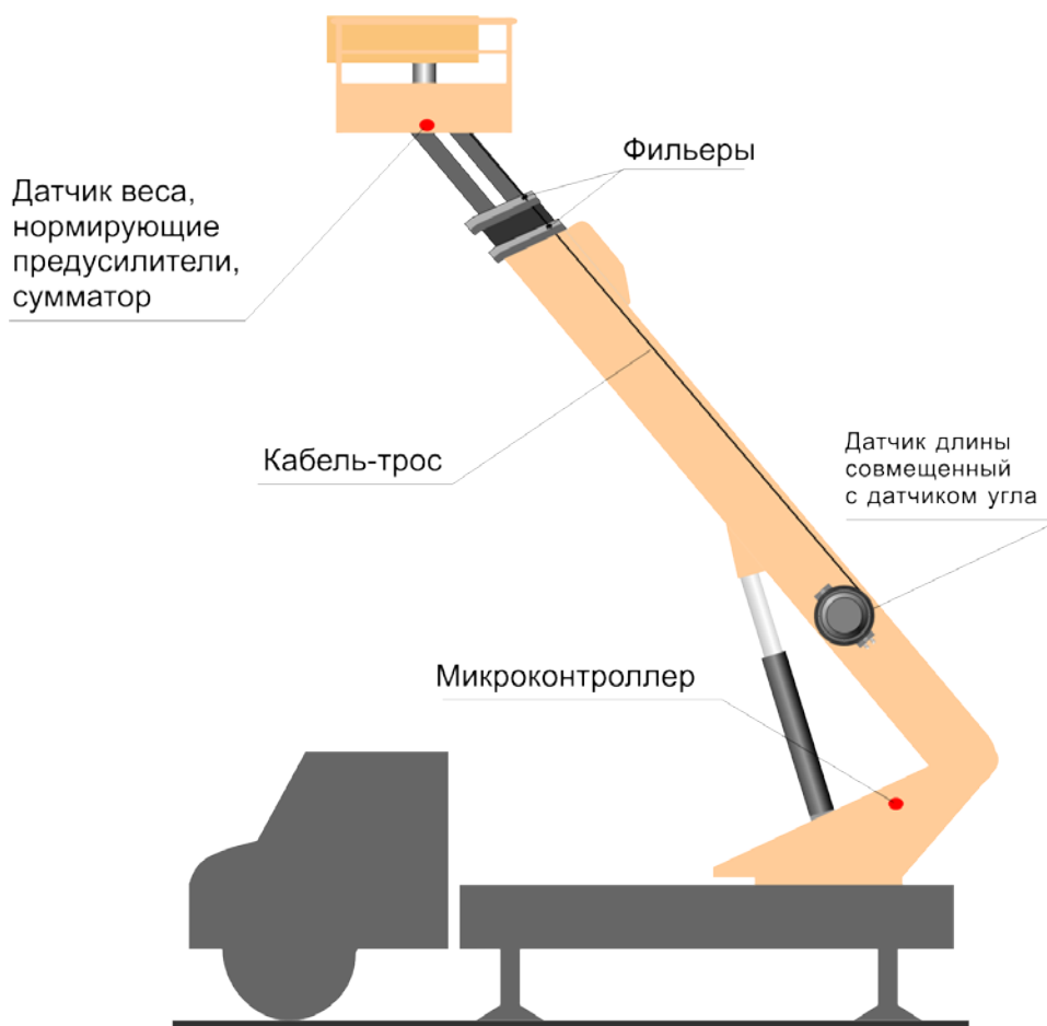
Рис.1 Система АС-АОГ-01м+ и ее размещение на подъёмнике
