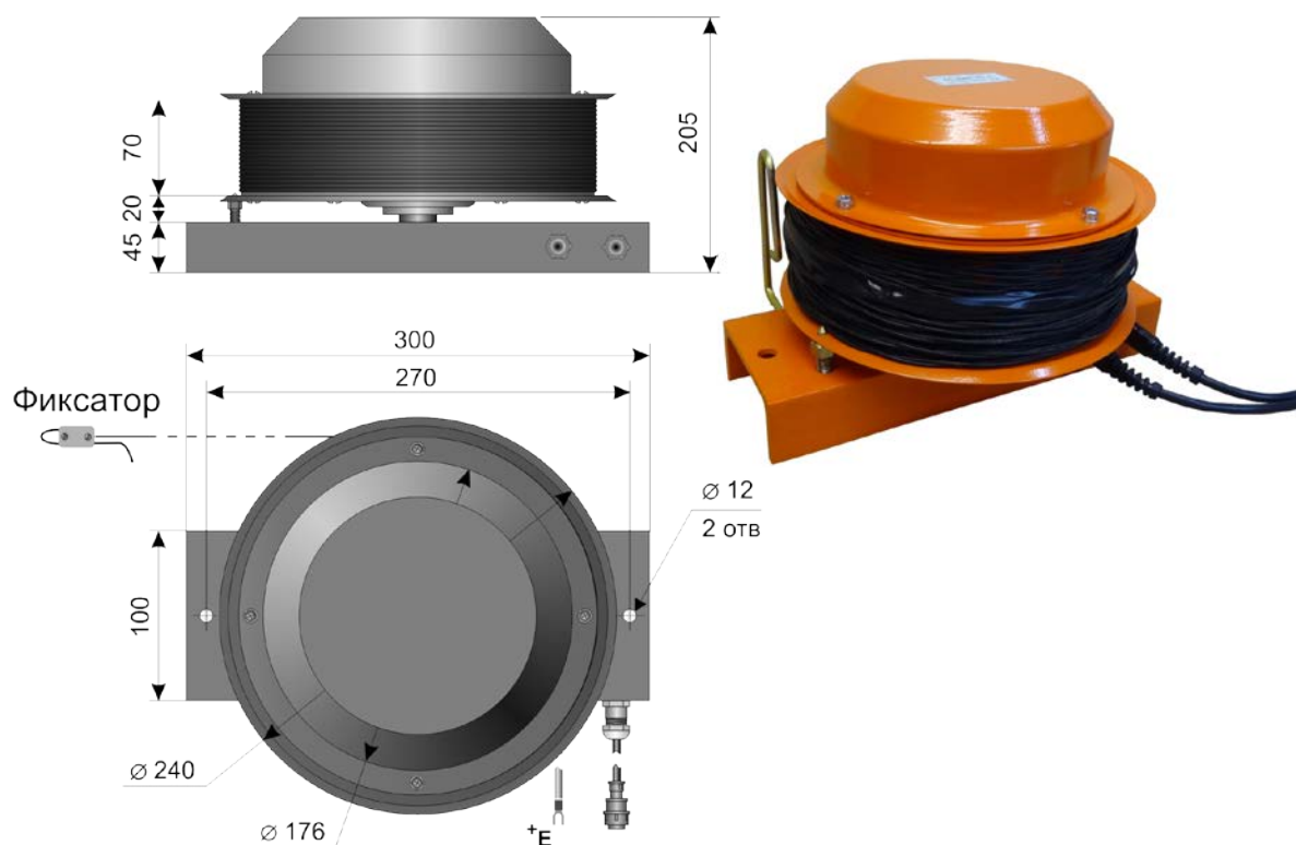
Рис.6 Датчик длины стрелы системы АС-АОГ-01м +
